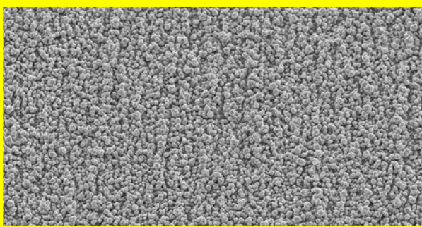
12µm treated-side Foil SEM × 1500
